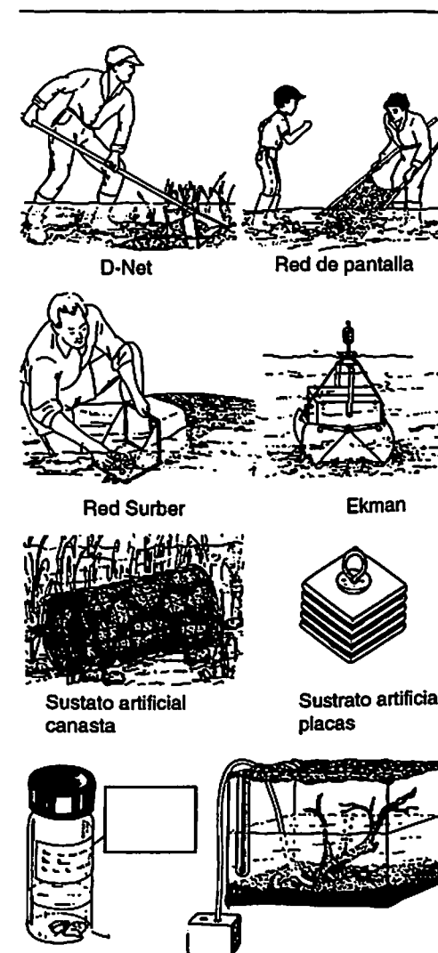
Figura 18.7 Métodos de recolección de macroinvertebrados acuáticos
