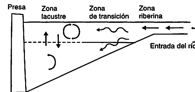
Figura 7.7 Zonas de un embalse
