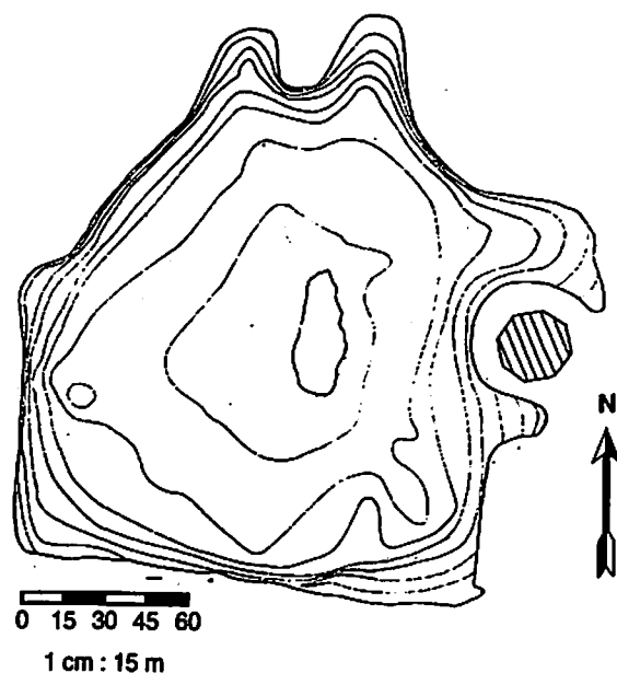
Figura 4.22 Mapa batimétrico de la laguna del Parque Norte
