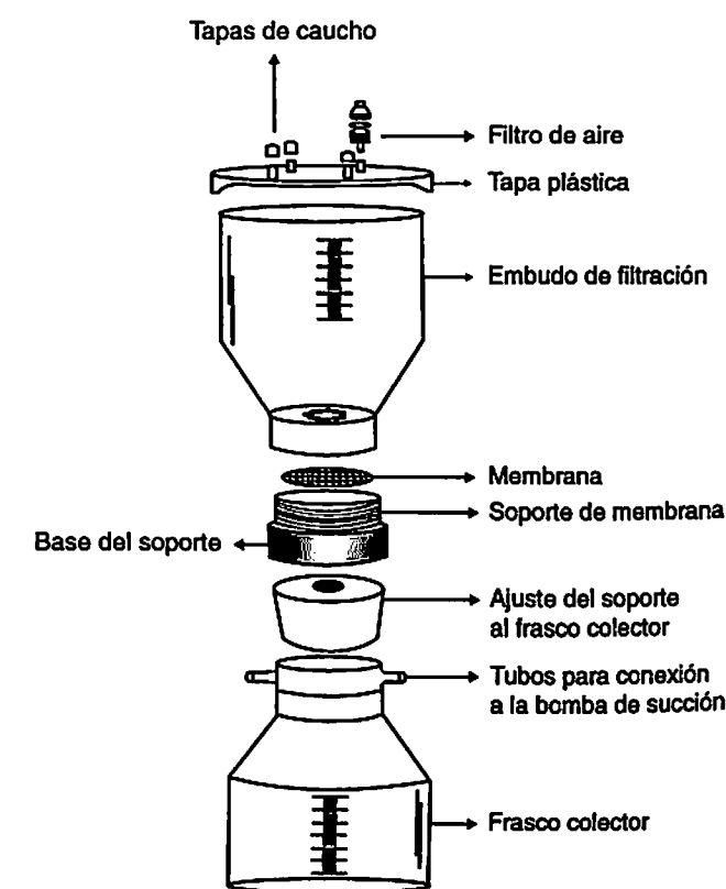
Figura 20.1 Componentes de un equipo de filtro de membrana
