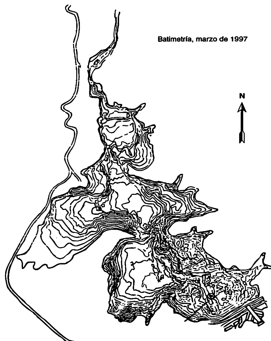
Figura 4.21 Mapa batimétrico de la represa La Fe, El Retiro (Colombia)
