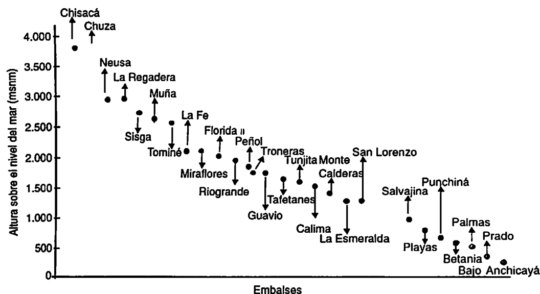
Figura 7.10 Distribución altitudinal de algunos embalses aprovechados para generar energía hidroeléctrica en Colombia
