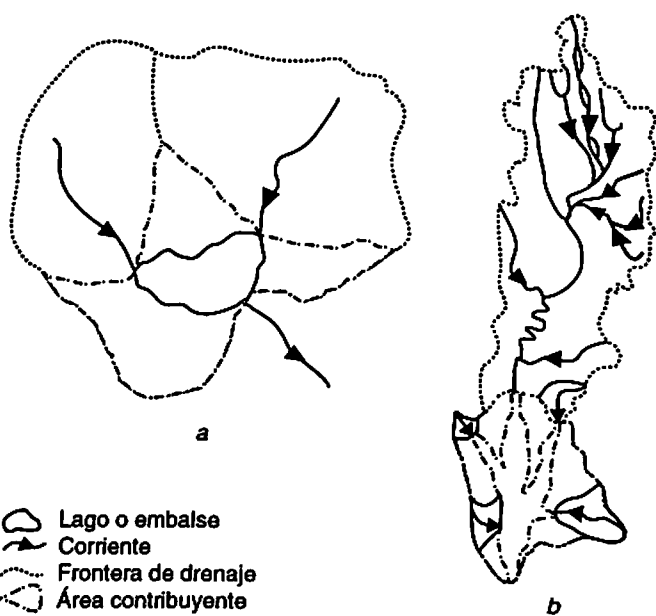
Figura 7.4 Características de la cuenca de drenaje. a. Lago; b. embalse.
