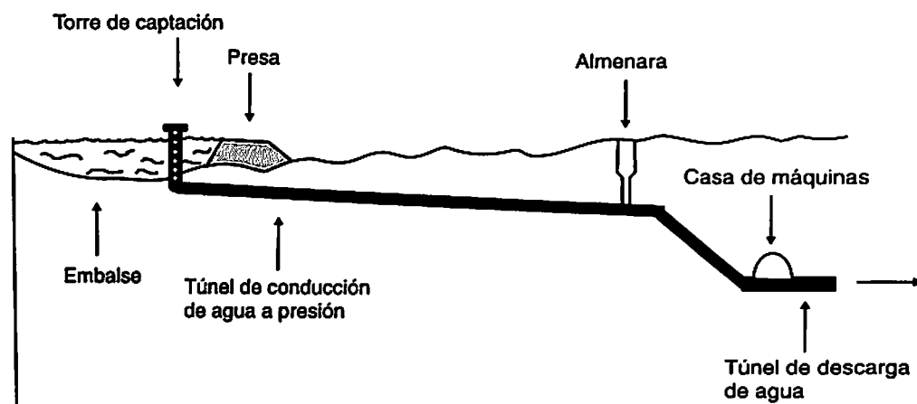
Figura 7.6 Perfil de un embalse con central hidroeléctrica
