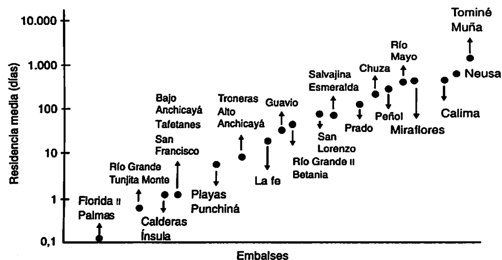
Figura 7.12 Tiempo de residencia en días de los principales embalses aprovechados para generar energía hidroeléctrica en Colombia
