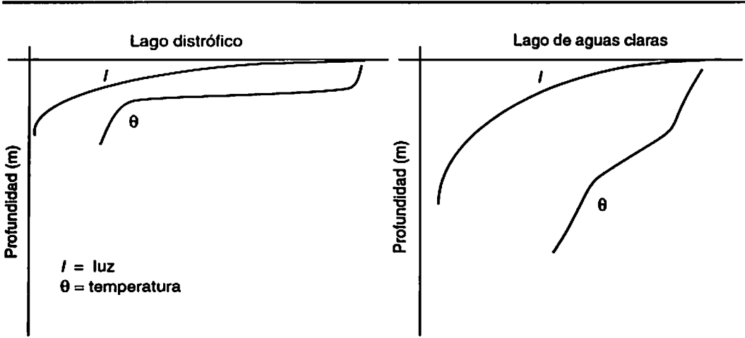
Figura 11.6 Variación vertical de la temperatura y la radiación en lagos de distinto estado trófico
