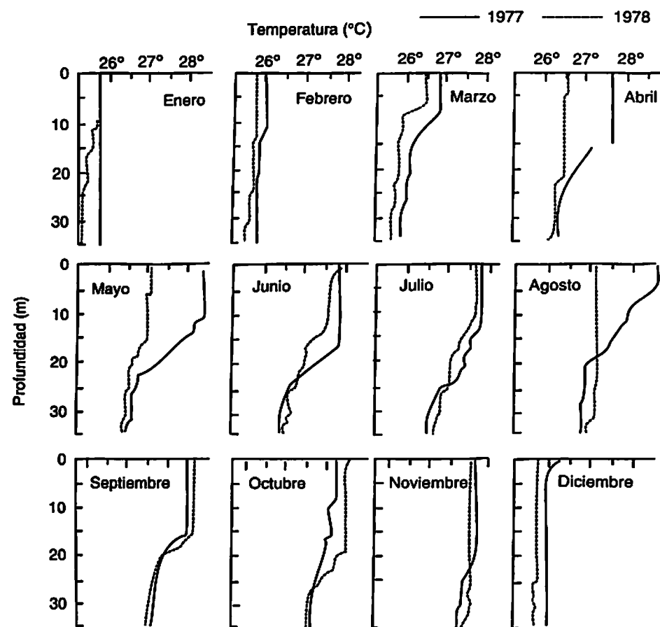
Figura 8.21 Perfiles de temperatura en la última semana de cada mes en el lago Valencia, Venezuela
