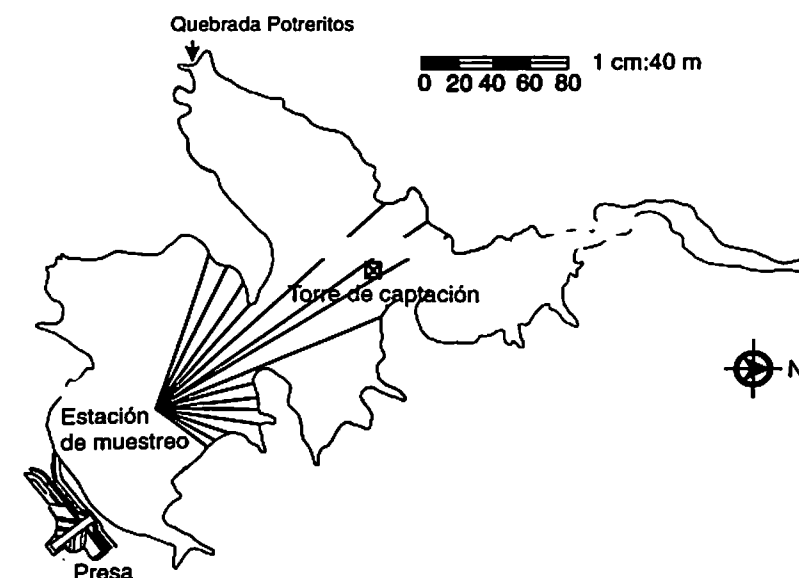
Figura 4.25 Mapa de la represa La Fe; obsérvese la manera de obtener el valor fetch
