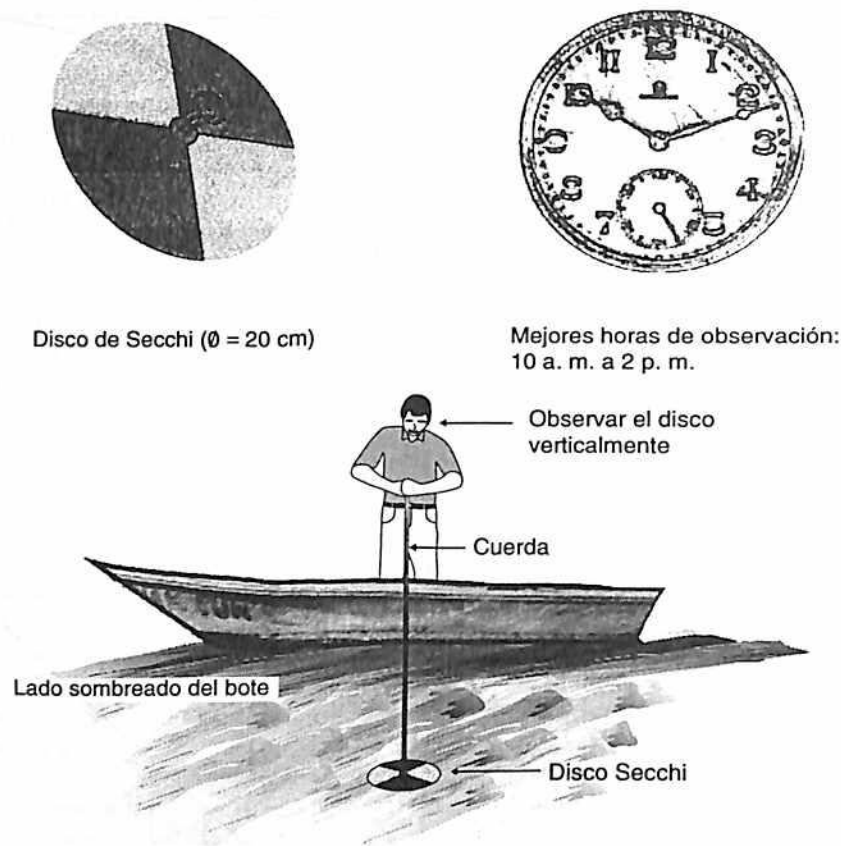
Figura 8.10 Forma y tiempo de medir la transparencia del agua con el disco Secchi
