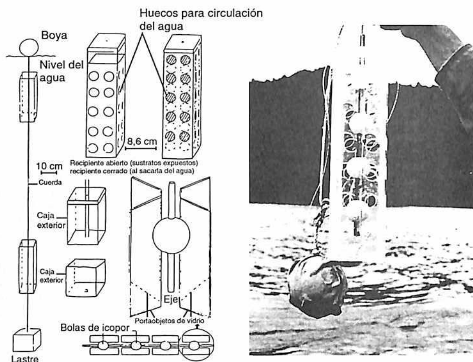
Figura 15.2 Muestreador para perifiton. a. Esquema (modificado de Lucey et al. , 1987); b. foto del muestreador en el campo.
