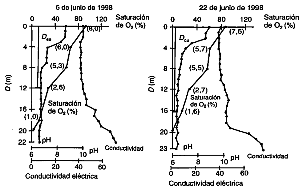
Figura 10.4 Variación vertical del porcentaje de saturación de \text{O}_2 , el pH y la conductividad durante junio de 1998 en la presa del embalse La Fe de El Retiro, Antioquia (Colombia)
