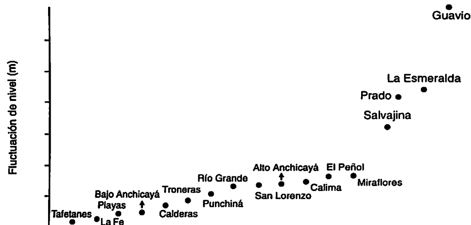
Figura 7.14 Fluctuaciones de nivel de algunos embalses aprovechados para generar energía hidroeléctrica en Colombia
