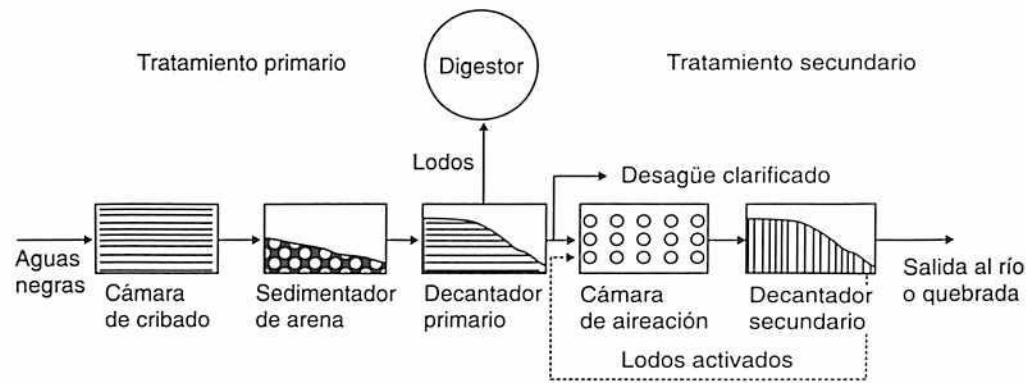
Figura 19.8 Tratamiento de aguas residuales por lodos activados
