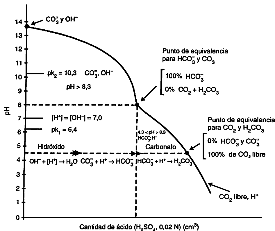
Figura 10.5 Curva de titulación de la alcalinidad
