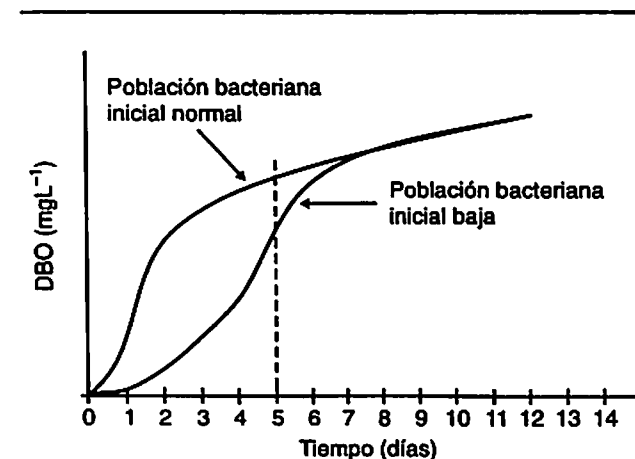
Figura 9.11 Efecto de una población bacteriana de baja densidad numérica en la DBO
