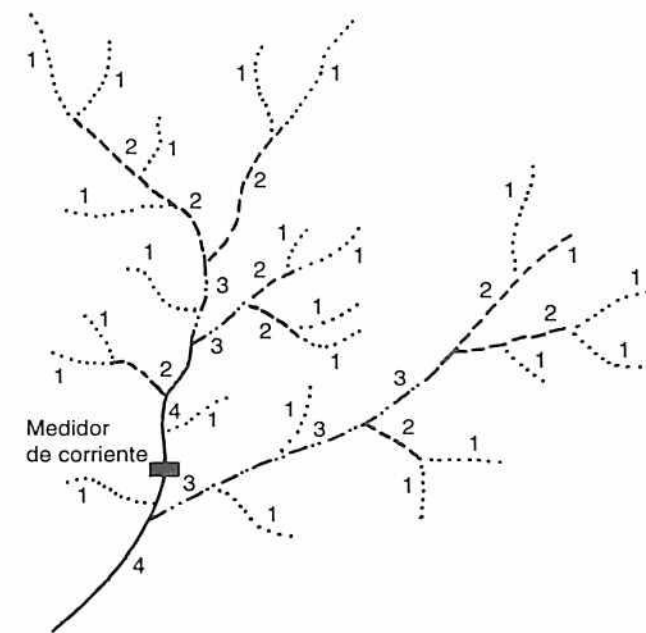
Figura 5.3 Red de drenaje que ilustra el orden de clasificación de corrientes para una cuenca de cuarto orden
