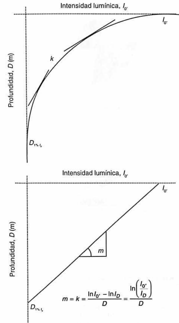
Figura 8.9 Atenuación exponencial de la luz y transformación logarítmica para hallar el valor del coeficiente de extinción k
