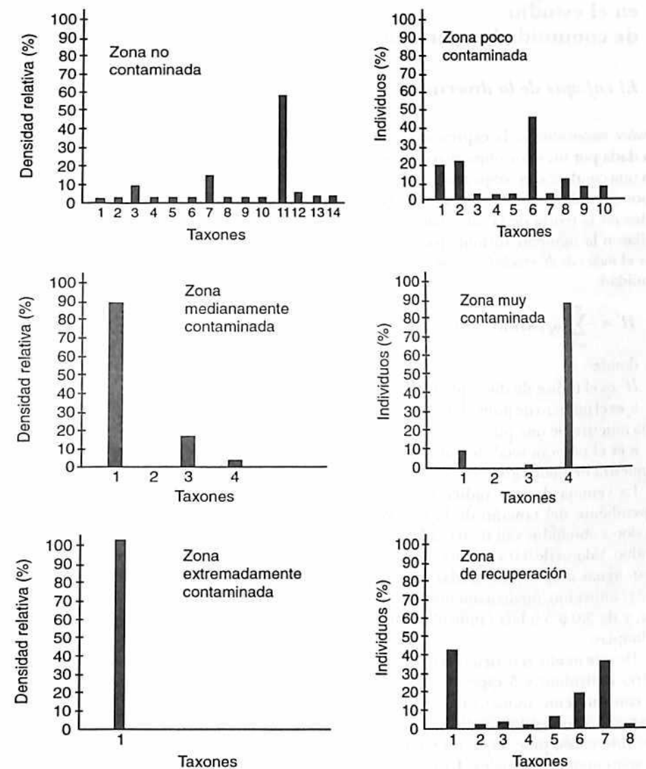
Figura 19.6 Modificación de las comunidades bentónicas en el río Medellín debido a la contaminación
