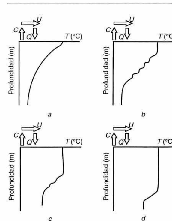
Figura 8.14 Variación diaria idealizada del perfil térmico en función de la entrada de calor ( Q ), el viento ( U ) y la convección ( C )
