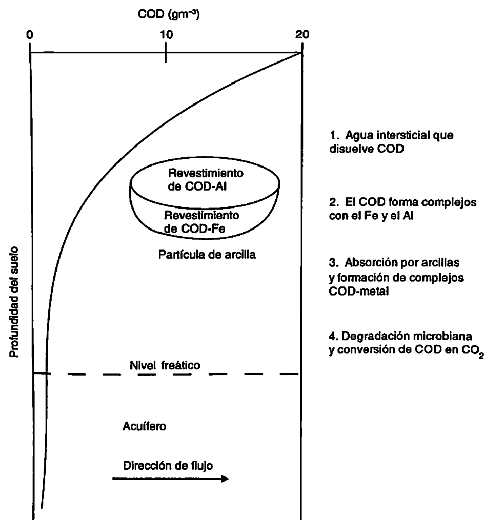
Figura 11.5 Disminución del COD en las aguas intersticiales del suelo
