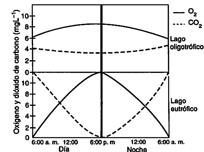
Figura 9.4 Representación idealizada de la variación de oxígeno y \text{CO}_2 en el ciclo día noche en un lago oligotrófico y uno eutrófico
