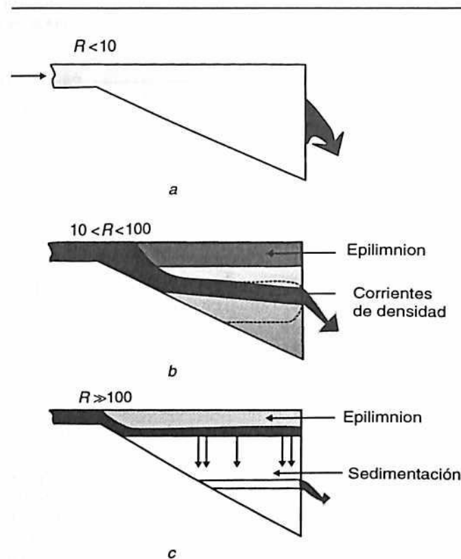
Figura 7.16 Representación del efecto de la variación en el tiempo de residencia en un embalse hipotético. a. Tiempo de residencia menor que 10 días; b. tiempo de residencia entre 10 y 100 días; c. tiempo de residencia de más de 100 días.
