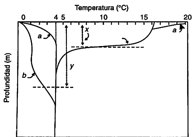
Figura 8.15 Tipos de termoclina. a: De superficie; b: de profundidad; x y y: altura del epilimnion.
