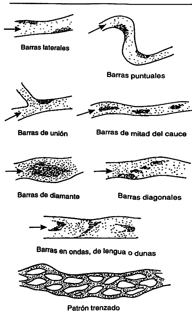
Figura 5.6 Clasificación morfológica de los grandes cauces: almacenamiento de sedimentos en barras
