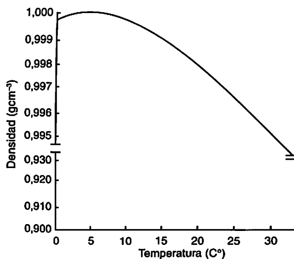
Figura 2.2 Relación entre temperatura y densidad del agua pura
