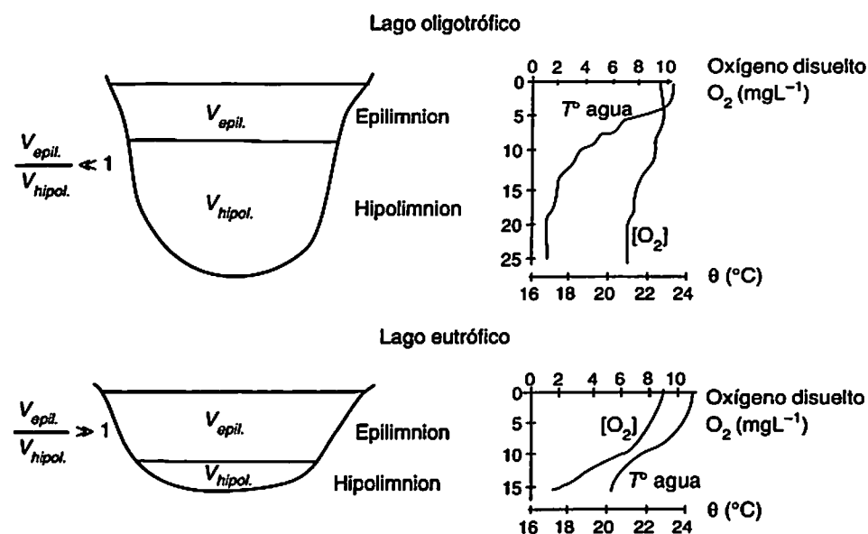
Figura 9.10 Volumen hipolimnético de oxígeno disponible para la degradación de la materia orgánica en lagos oligotróficos y eutróficos
