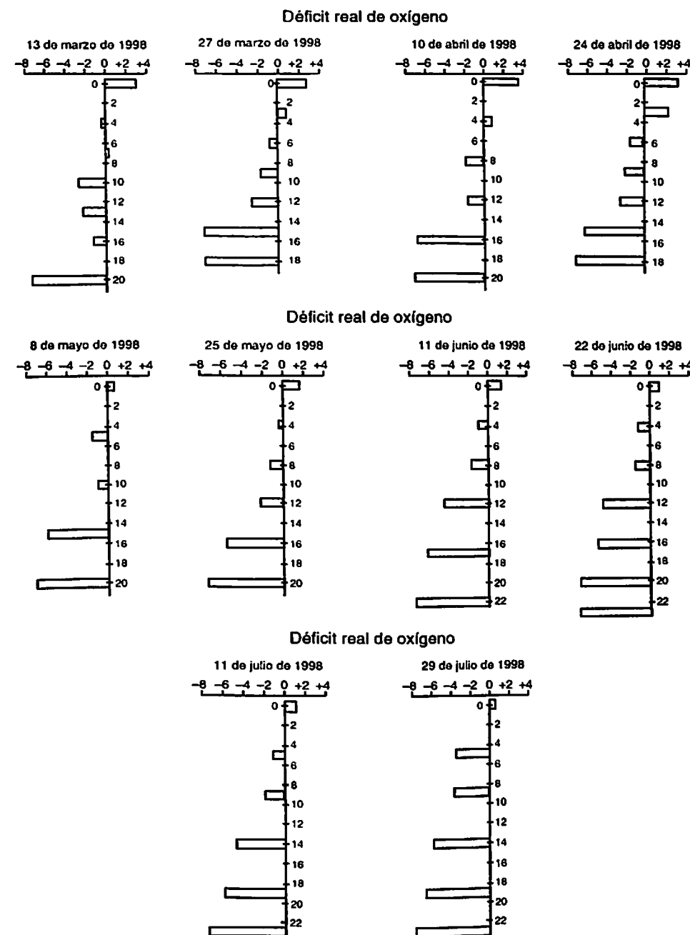
Figura 9.7 Valores del déficit real de oxígeno entre marzo y julio de 1998 en la represa La Fe, Antioquia (Colombia).
