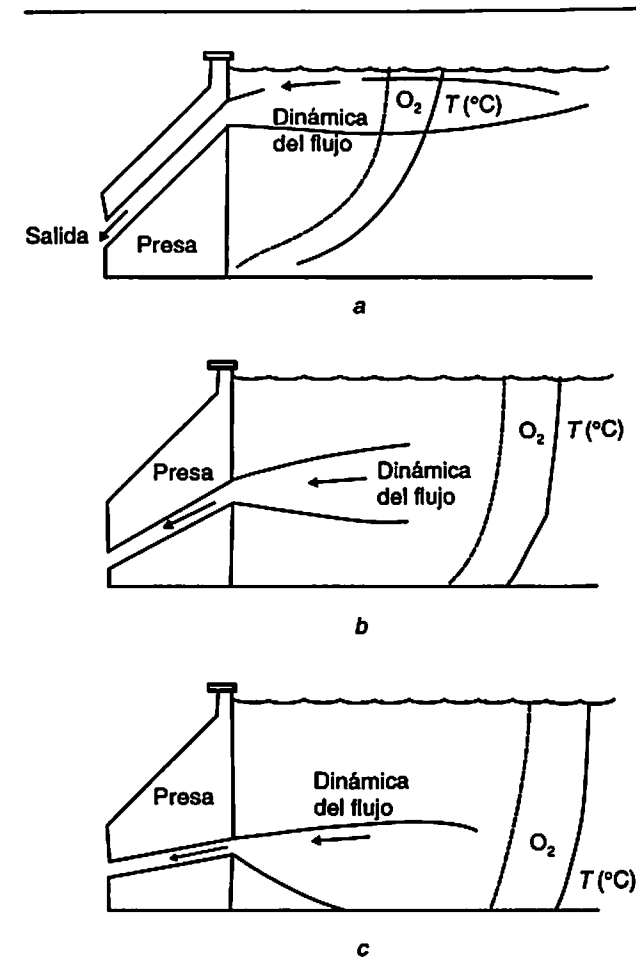
Figura 7.17 Tipos de salida de algunos embalses. a. Embalse exportador de calor, de aguas cálidas y pobres en nutrientes. b. Embalse con salida media de agua de menor temperatura. c. Embalse con salida baja de agua fría con altas concentraciones de nutrientes.
