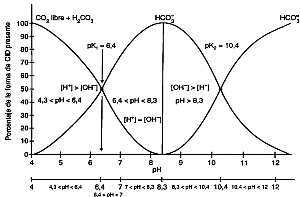
Figura 10.1 Variación del porcentaje de las formas del CID frente a los cambios de pH
