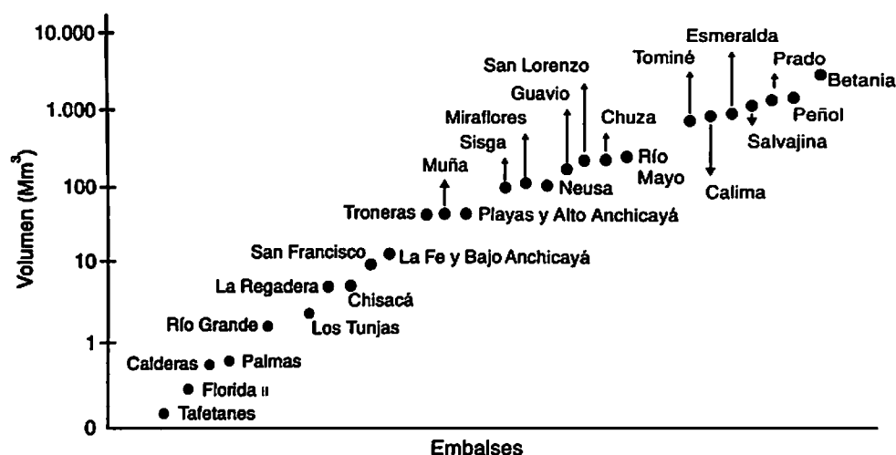
Figura 7.15 Volumen total de algunos embalses aprovechados para generar energía hidroeléctrica en Colombia
