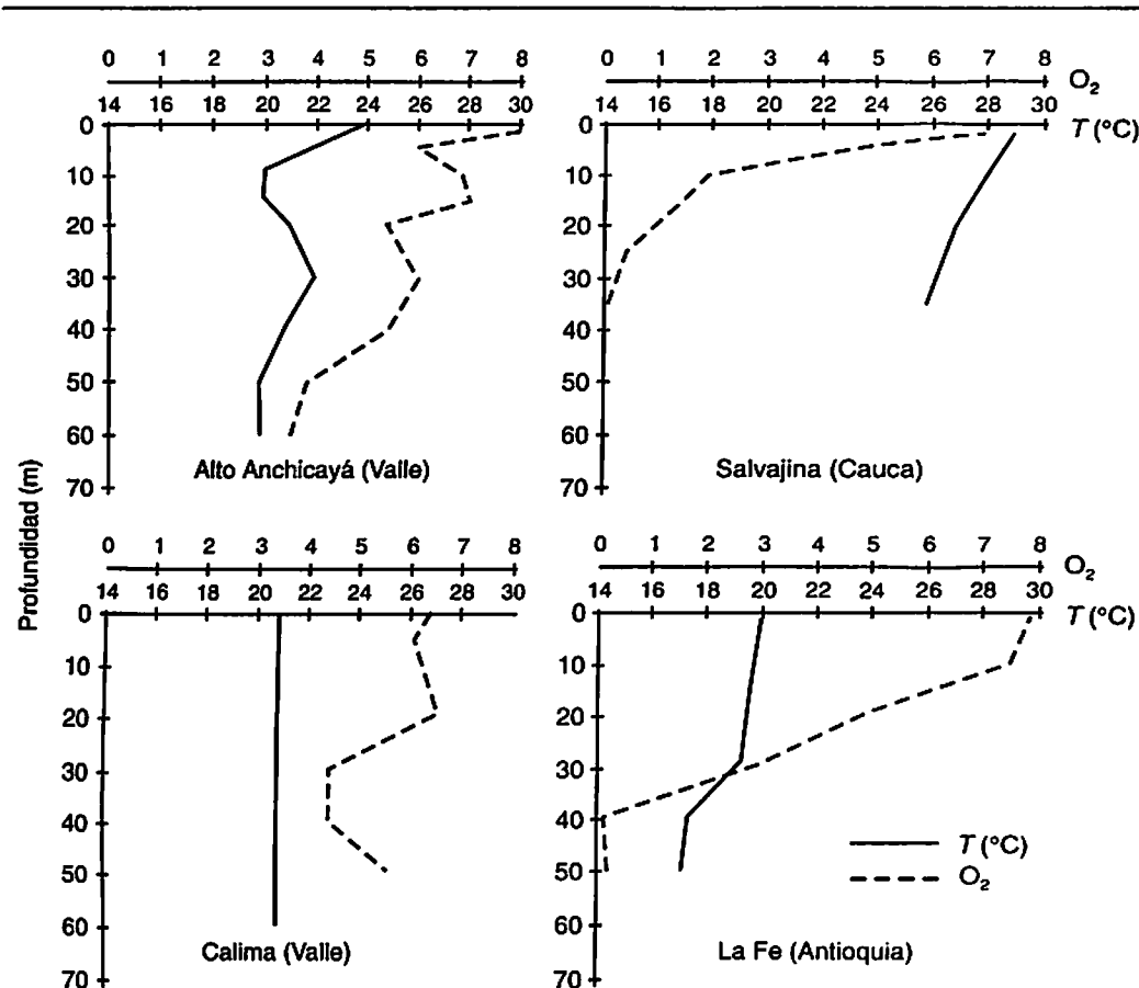
Figura 7.18 Perfiles de temperatura y oxígeno en cuatro embalses colombianos. Alto Anchicayá y Calima muy mezclados; Salvajina y La Fe muy estratificados.
