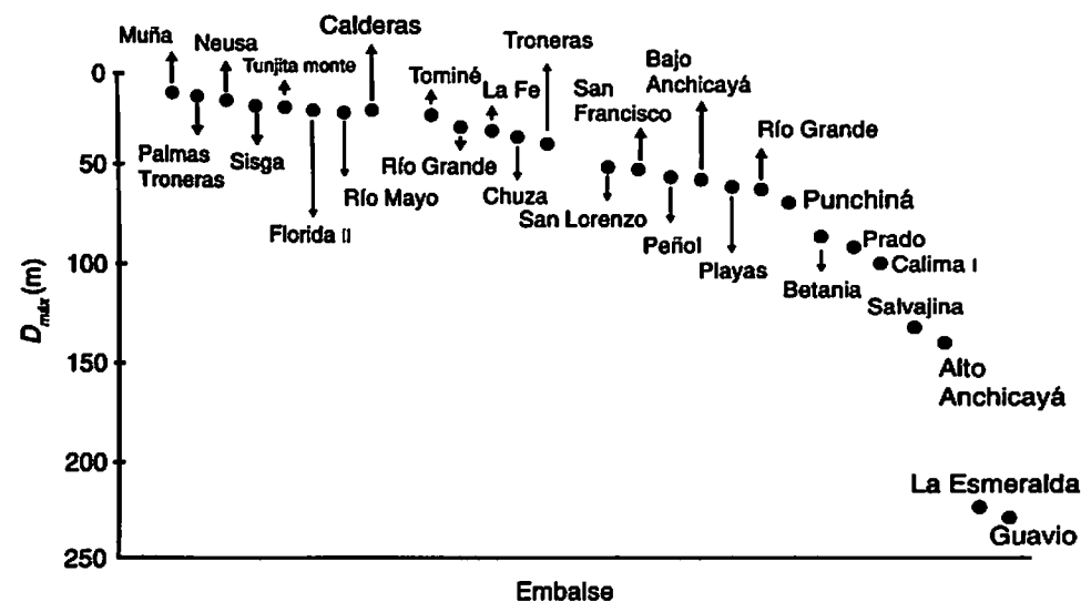
Figura 7.13 Profundidades máximas de algunos embalses aprovechados para generar energía hidroeléctrica en Colombia
