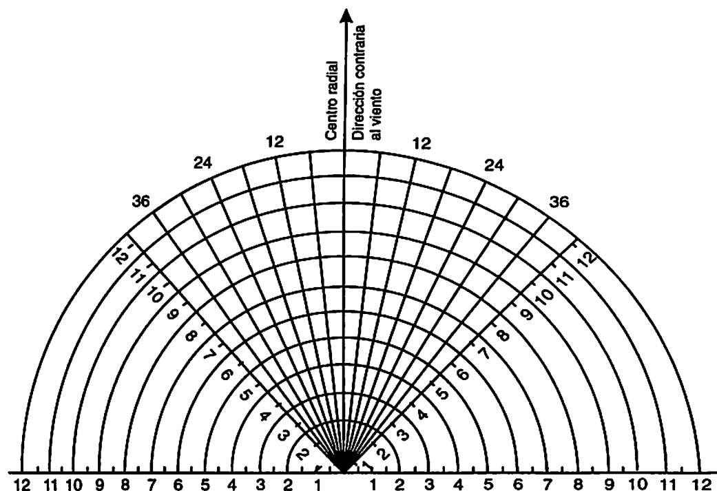
Figura 4.24 Herramienta gráfica diseñada por el Beach Erosion Board para obtener el valor de fetch
