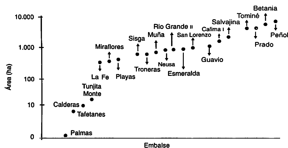
Figura 7.11 Área del espejo de agua de algunos embalses aprovechados para generar energía hidroeléctrica en Colombia
