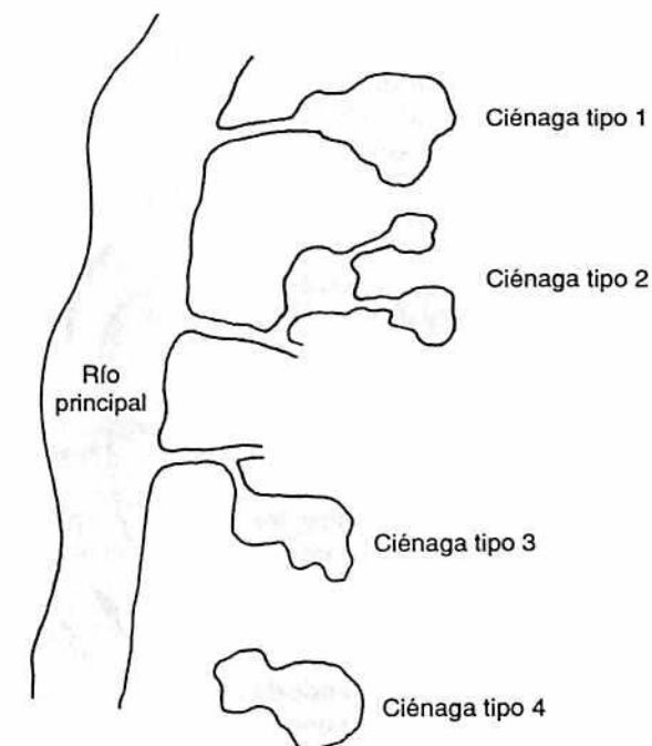
Figura 4.18 Tipos de ciénagas de origen fluvial
