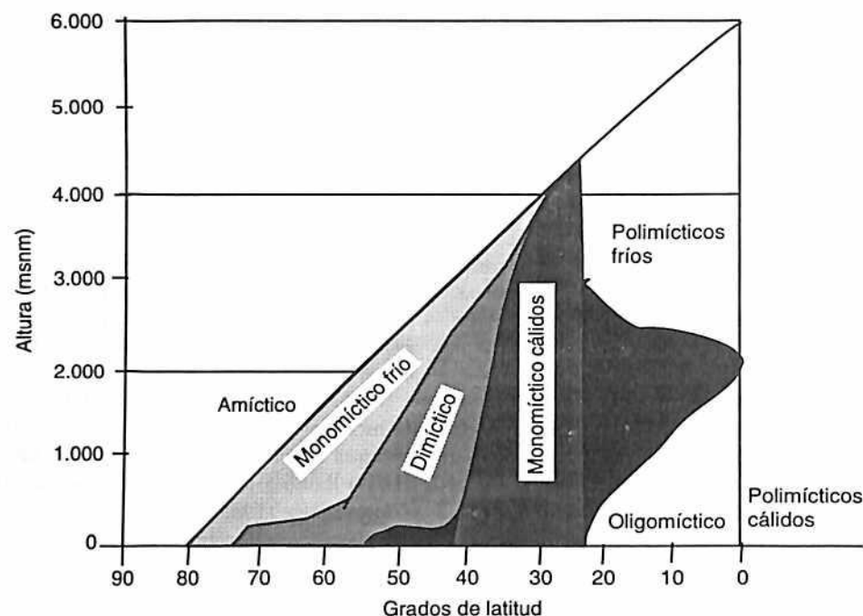
Figura 8.22 Representación esquemática de acuerdo con la clasificación térmica de los lagos organizados según latitud y altitud
