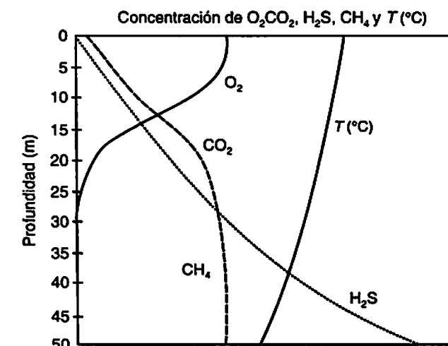
Figura 9.3 Comportamiento vertical de algunas variables químicas y de la temperatura en un embalse con vegetación inundada
