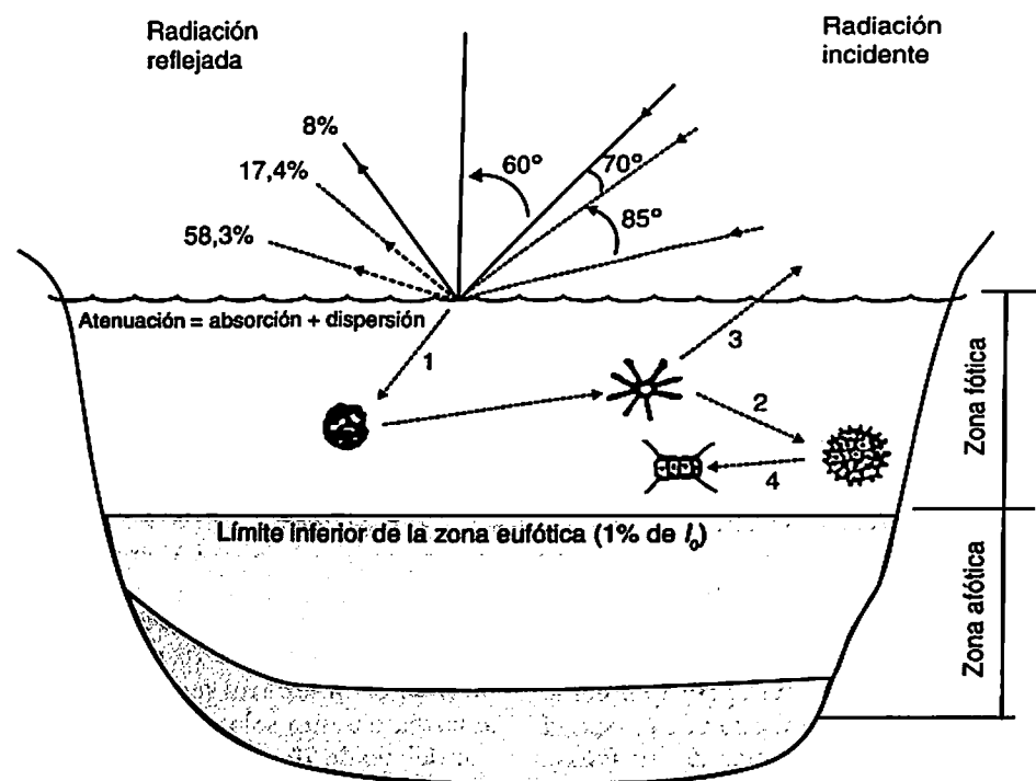
Figura 8.4 Atenuación de luz incidente al penetrar en la columna de agua
