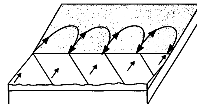
Figura 4.12 Desplazamiento de arenas a lo largo de la playa cuando las olas baten oblicuamente
