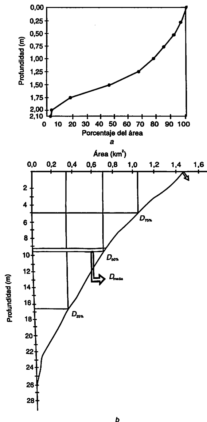
Figura 4.27 Curvas hipsográficas. a. Laguna del Parque Norte; b. Represa La Fe.
