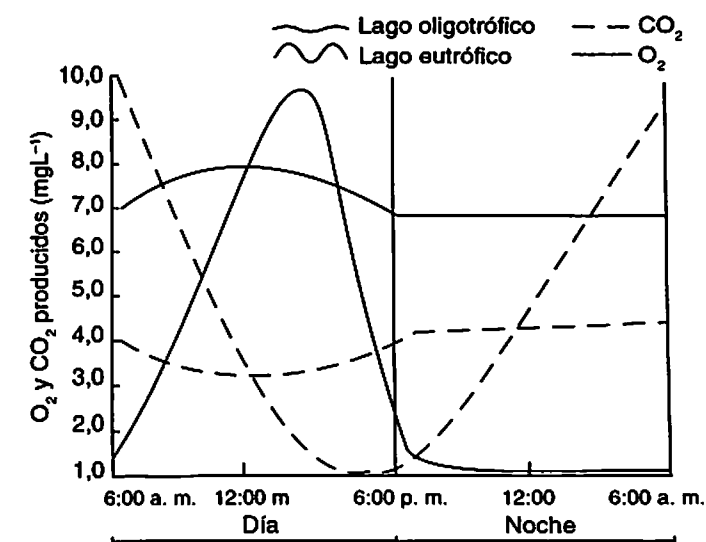
Figura 2.17 Variación de concentraciones de O_2 y CO_2 en el ciclo día-noche en un lago oligotrófico y en uno eutrófico
