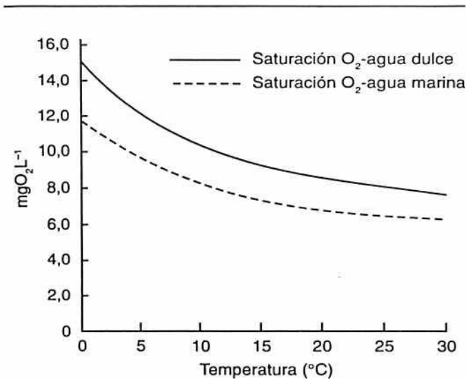
Figura 2.18 Curvas de saturación de oxígeno a diferentes temperaturas en aguas dulce y marina
