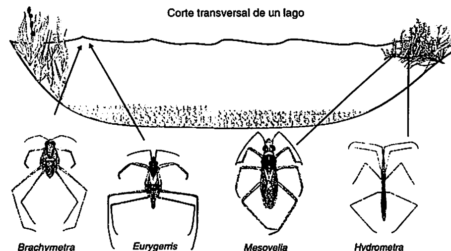
Figura 18.2 Organismos representativos del neuston en un ecosistema de lago
