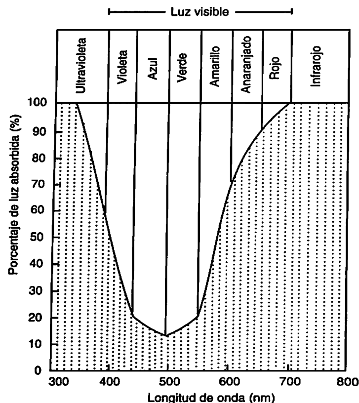
Figura 2.16 Absorción de luz en una columna de agua pura y penetración diferencial de las distintas longitudes de onda
