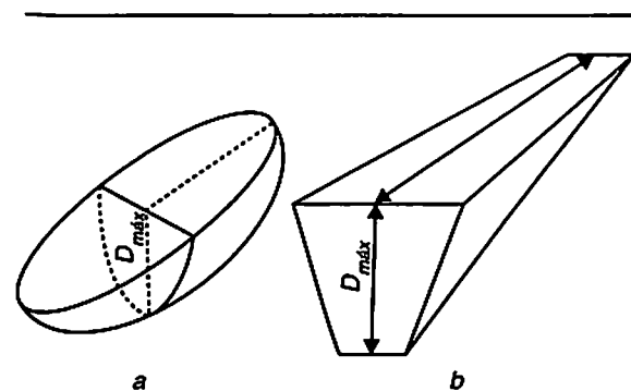
Figura 7.3 Representación simplificada de morfometrías. a. un lago. b. un embalse
