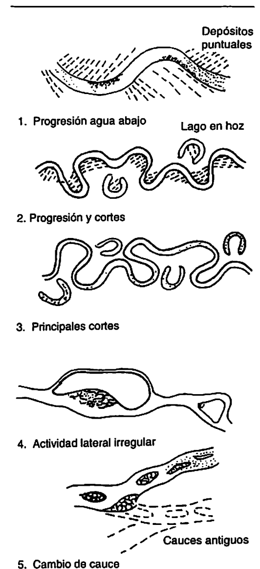
Figura 5.7 Actividad lateral de los grandes cauces
