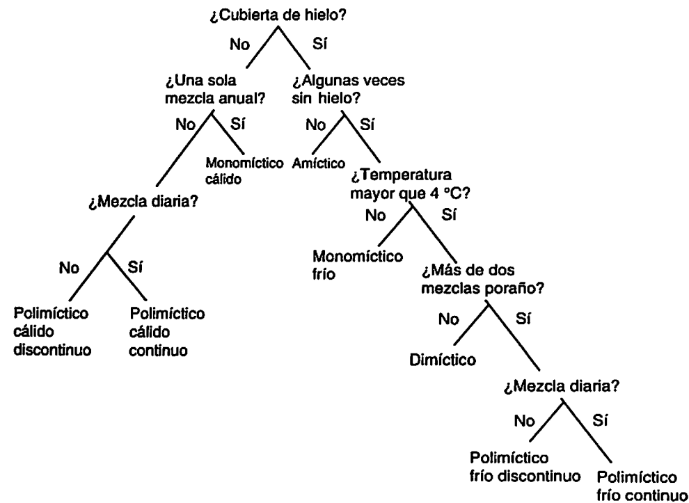
Figura 8.23 Clave dicotómica para clasificar lagos según su patrón de mezcla
