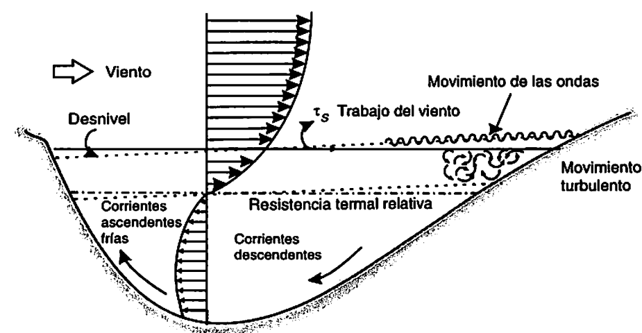
Figura 8.12 Esquema general del intercambio de energía mecánica en la interfase aire-agua como proceso básico en la hidrodinámica de lagos holomícticos
