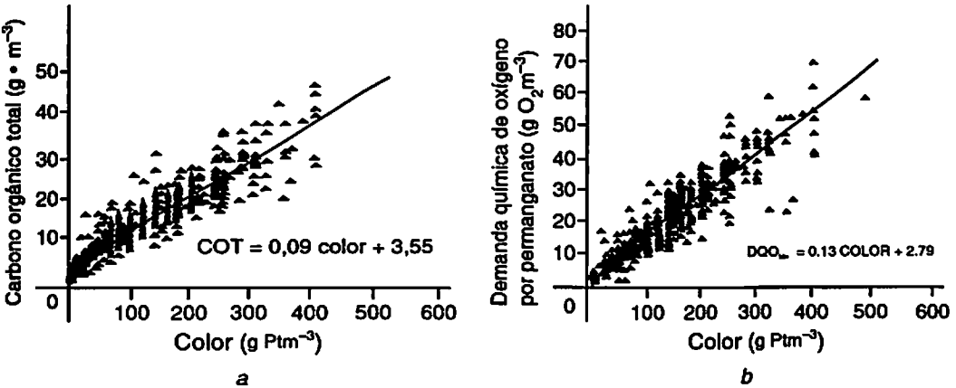
Figura 11.7 Relación entre el color del agua y las concentraciones de COT y DQO
