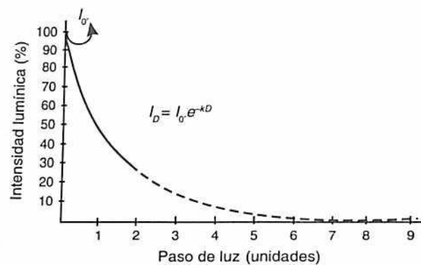
Figura 8.8 Atenuación exponencial de la radiación superficial ( I_0 ) con la profundidad
