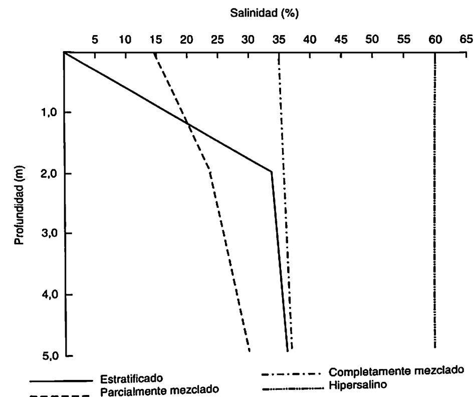
Figura 6.6 Tipos de estuarios de acuerdo con la clasificación salina y los patrones de circulación
