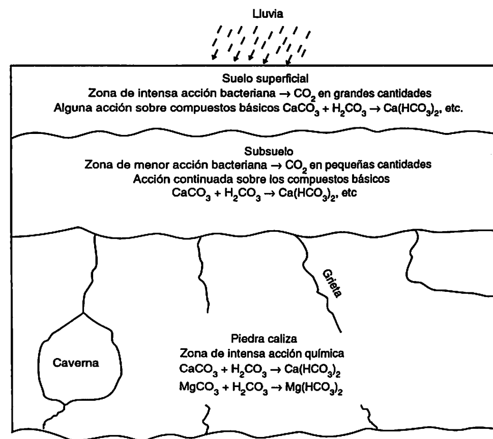
Figura 12.1 Fuentes de \text{CO}_2 y la solución de las sustancias causantes de la dureza
