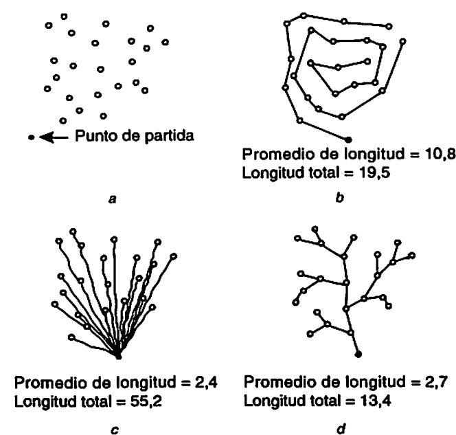
Figura 5.9 Comparación teórica de eficiencia de patrones de drenaje. a. Drenaje a través de un punto de partida; b. Drenaje en espiral; c. Configuración tipo explosión; d. Patrón ramificado. Las medidas se dan en unidades arbitrarias.
