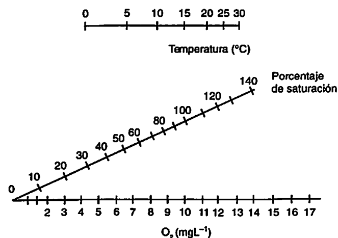
Figura 9.2 Forma de determinar el porcentaje de saturación de oxígeno a partir de la temperatura del agua y la concentración de oxígeno medida
