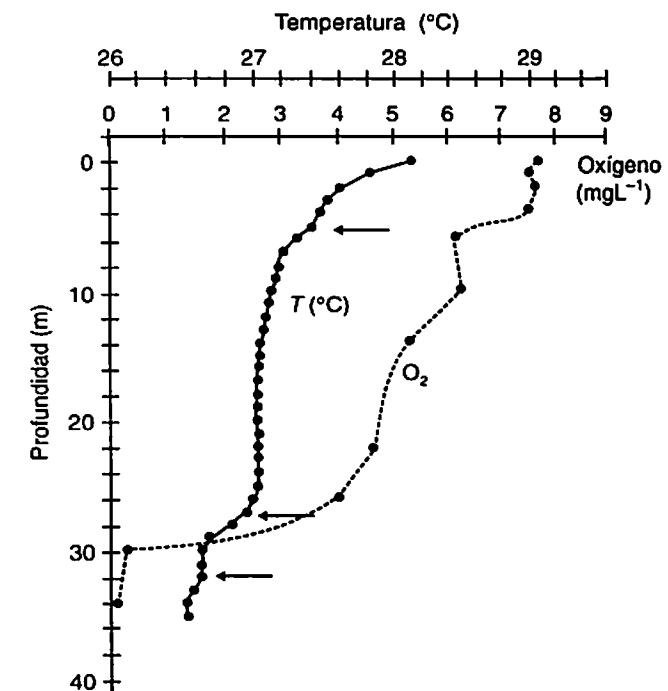
Figura 8.24 Termoclinas múltiples (indicadas por flechas) en el Lago Valencia, Venezuela
