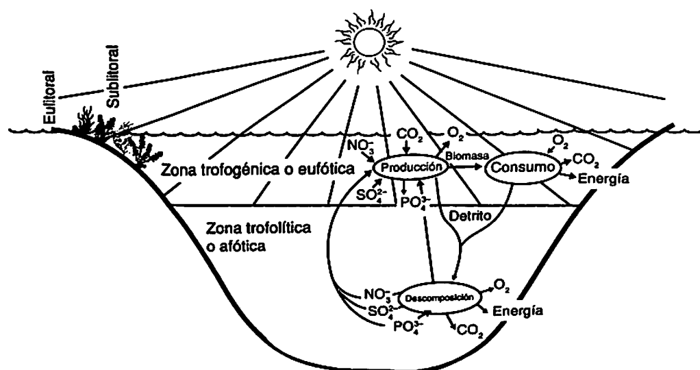
Figura 2.21 Principales etapas del metabolismo en un ecosistema acuático
