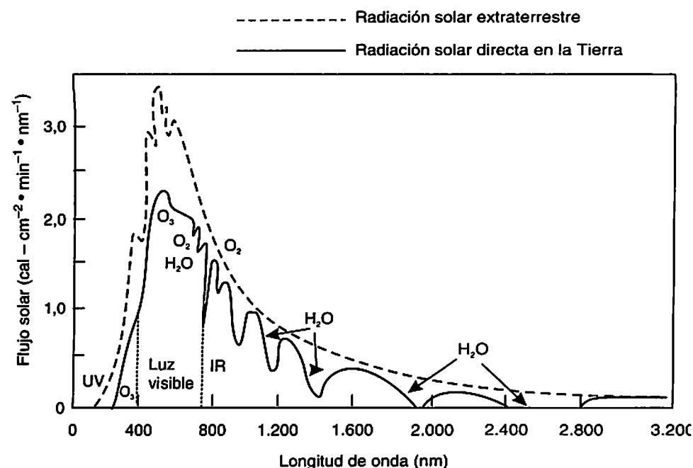
Figura 8.2 Radiación solar extraterrestre y la que cae directamente sobre la Tierra; se muestran las principales bandas de absorción de oxígeno, ozono y vapor de agua.
