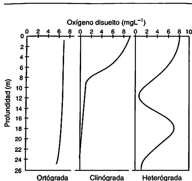
Figura 9.5 Tres tipos de perfiles de oxígeno que pueden presentarse en lagos y embalses
